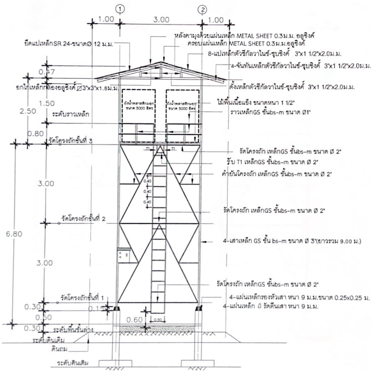
รูปตัด มาตรฐาน 1:50
