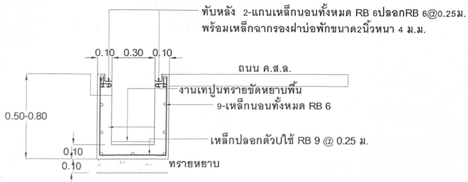
รูปตัดฝารางระบายน้ำ ค.ส.ล.
