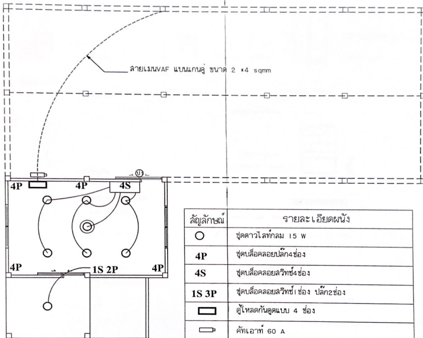
แปลนไฟฟ้า
