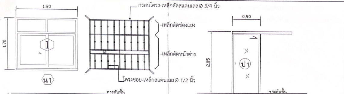
รายละเอียดเพิ่มเติมมาติดตั้งใหม่จำนวน 2 ชุด พร้อมติดตั้งเหล็กตัดสแตนเลสแบบครอบ) ๗๑
