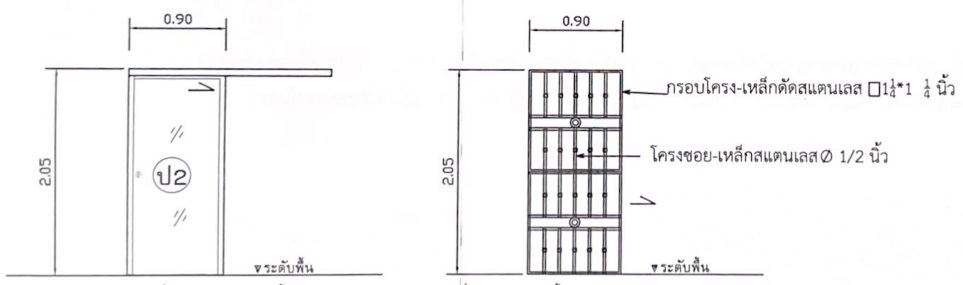
ประตูกระจกบานเลื่อน 1 ชุด พร้อมติดตั้งประตูเหล็กสแตนเลสแบบบานเลื่อน 1 ชุด (ติดตั้งทางออกระเบียง)
