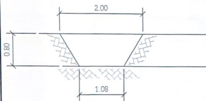
รูปตัดคูเดิม
