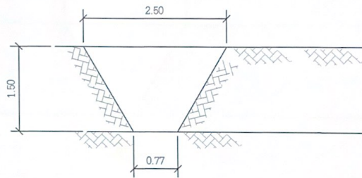
รูปตัดขุดลอกคูใหม่
