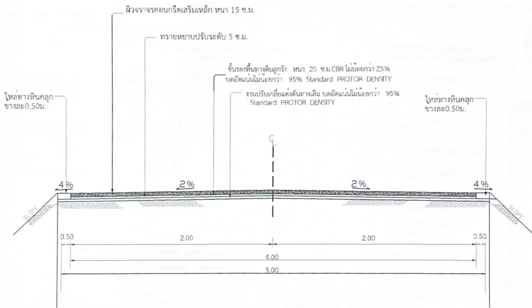
รูปตัดถนนคอนกรีตเสริมเหล็ก หนา 15 ซม. มาตรฐาน NO SCALE
