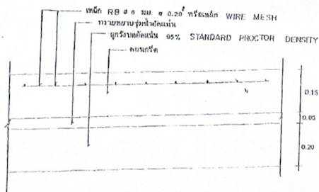
รายละเอียดขนาดของเหล็กเสริมเหล็ก
