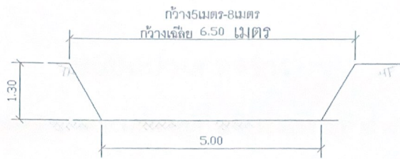
รูปตัดสภาพเดิม
