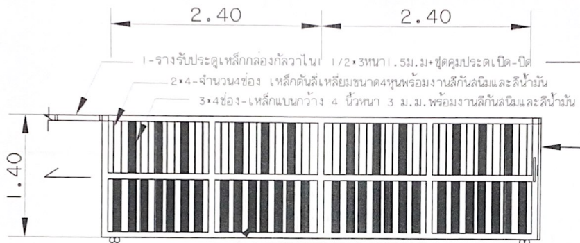
ขยายประตูรั้ว
