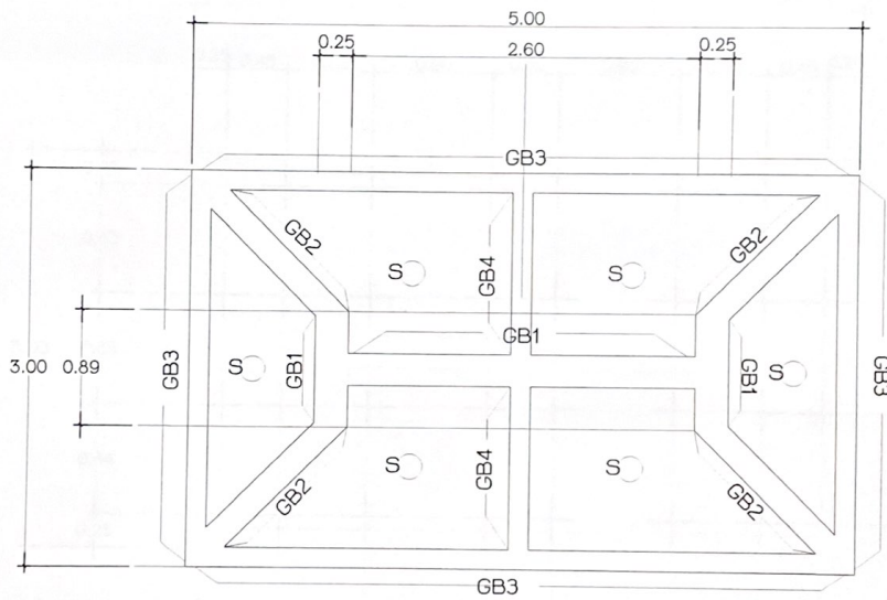
แปลนขยายคานคอดิน-พื้น มาตรฐาน 1:30
