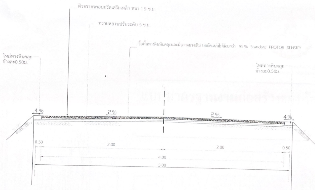
รูปตัดถนนคอนกรีตเสริมเหล็ก ทหนา 15 ซม.
