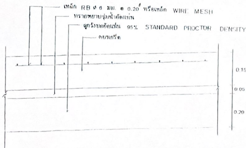
รายละเอียดงานคอนกรีตเสริมเหล็ก
