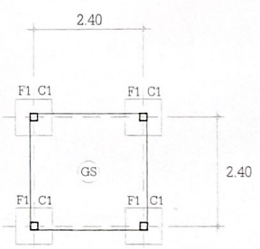
แผ่นพื้น F1,C1
