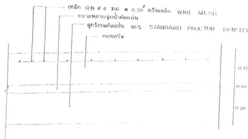
รายละเอียดขนาดและชนิดเหล็กเสริม
