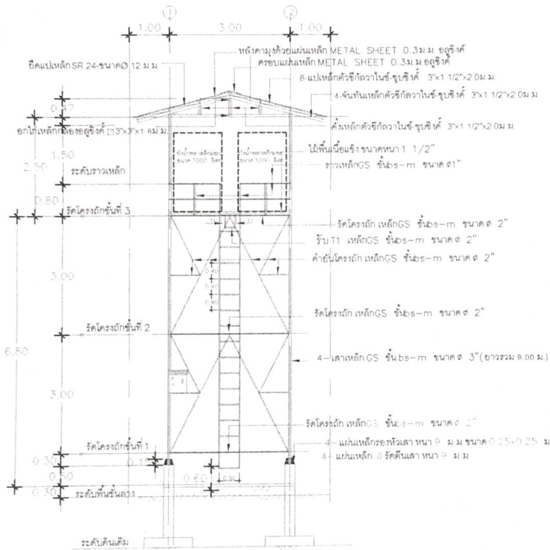
รูปตัด มาตราส่วน 1:50
