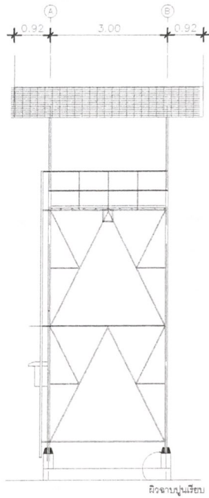
รูปด้าน 2 มาตราส่วน 1:50
