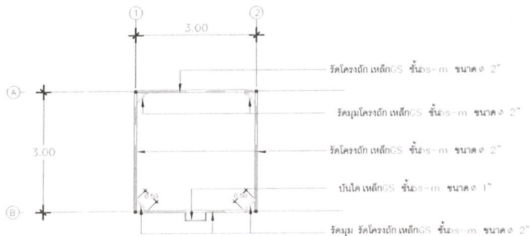
แปลนโครงสร้างเหล็กดัดที่ 1-2 มาตราส่วน 1:40
