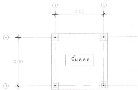
แปลนพื้น มาตราส่วน 1:40
