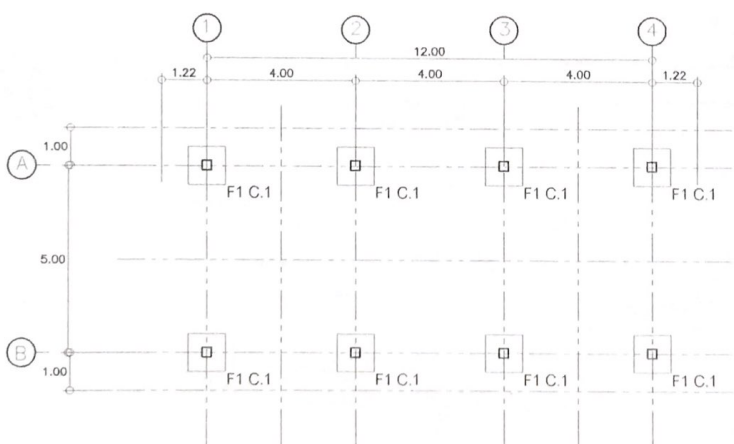
แปลนฐานราก ตอม่อ เสา มาตรฐาน ส่วน 1:75
